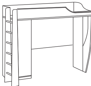
Кровать-чердак со шкафом "Дисней" Ш.2210 Г.852 В.1780
