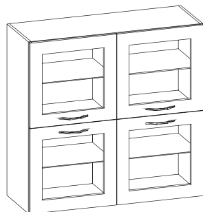
Шкаф 4-дверный навесной "Таис" Ш.1002 Г.370 В.970
