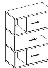
Стеллаж Ш.800 Г.375 В.1100
