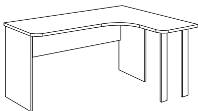
Стол угловой "Дисней" Ш.1420 Г.1160 В.750
