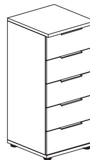
Комод 5 ящиков "Париж" Ш.510 Г.550 В.1120
