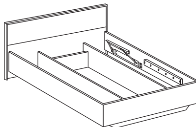
Кровать с подъемным основанием "Бостон" Матрац 1400*1950 Матрац 1200*1950 Матрац 900*1950
