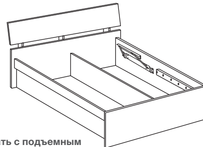
Кровать с подъемным основанием "Париж" Матрац 1400*1950 Матрац 1200*1950 Матрац 900*1950
