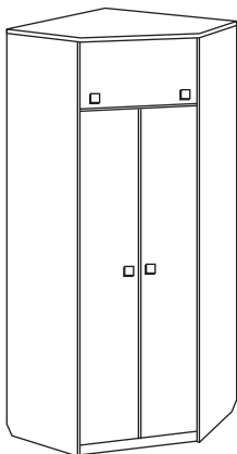
Шкаф угловой "Дисней" Ш.1000/900 Г.450/550 В.2204
