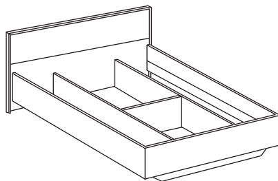
Кровать "Бостон" Матрац 1400*1950 Матрац 1200*1950 Матрац 900*1950
