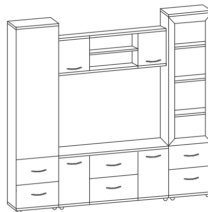
Стенка "Ялта" Ш.2400 Г.450 В.2100
