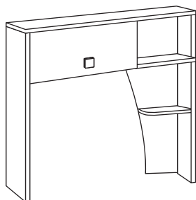
Полка стола 1140 "Дисней" Ш.1140 Г.300 В.1085
