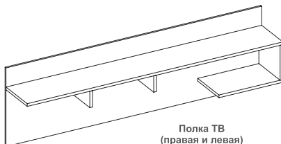
Полка ТВ (правая и левая) Ш.1800 Г.375 В.640
