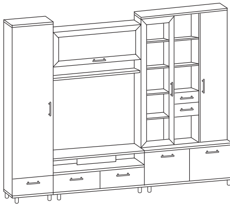
Стенка "Ника" Ш.2900 Г.520 В.2110
