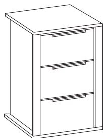
Секция с тремя ящиками Ш.430 Г.490 В.732
