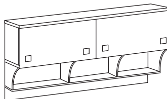
Полка навесная №2 "Дисней" Ш.2000 Г.320 В.780
