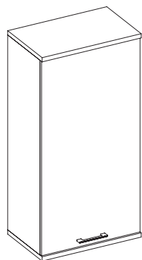
Шкаф подвесной (правый и левый) Ш.600 Г.375 В.1200
