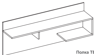
Полка ТВ (правая и левая) Ш.1800 Г.375 В.640
