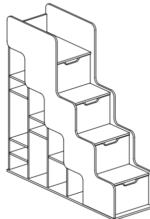
Лестница с ящиками "Дисней" Ш.1440 Г.450 В.1515
